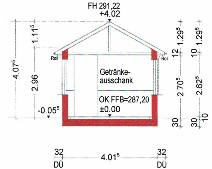
Schnitt 1-1
