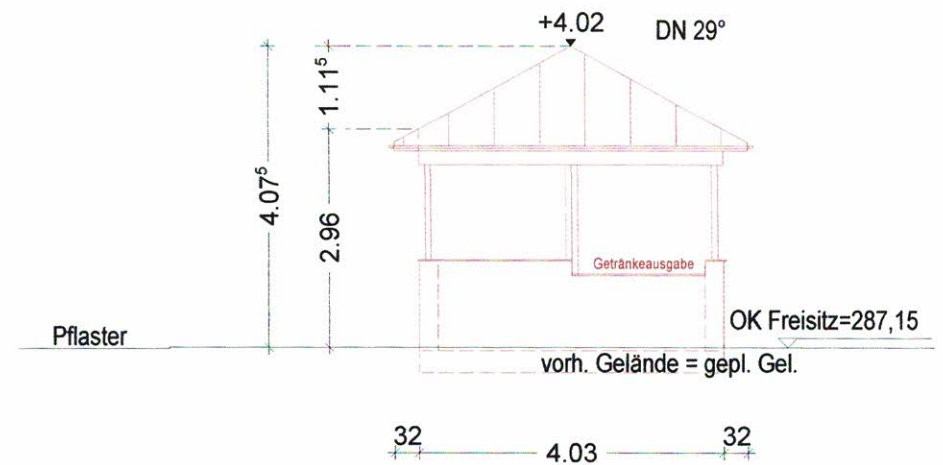
Ansicht Nord/Ost
